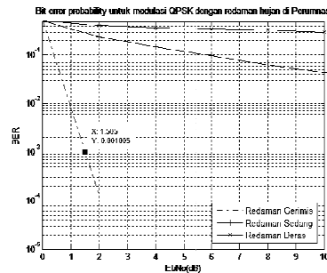
Gambar 9. Modulasi QPSK pada daerah Perumnas
