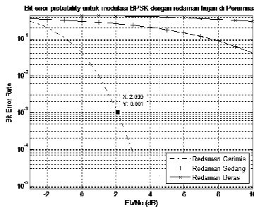
Gambar 8. Modulasi BPSK pada daerah Perumnas
