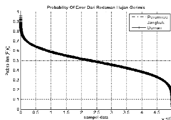
Gambar 10. Waterfilling dengan Probabilitas Redaman Hujan Gerimis
