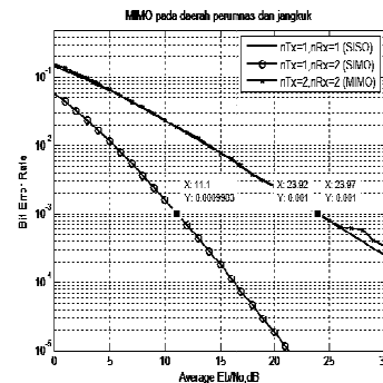
Gambar 7. MIMO Dengan Hujan Gerimis Pada Daerah Perumnas Dan Jangkuk
