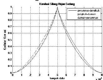
Gambar 6. Korelasi Silang Pada Hujan Sedang
